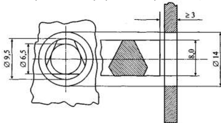
Размеры ключевины устройства отпирания замка, мм
