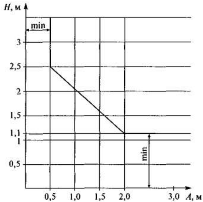
Рис. 2. Высота ограждения шахты в зависимости от расстояния до движущихся элементов лифта: А - расстояние до движущихся элементов лифта Н - высота ограждения
